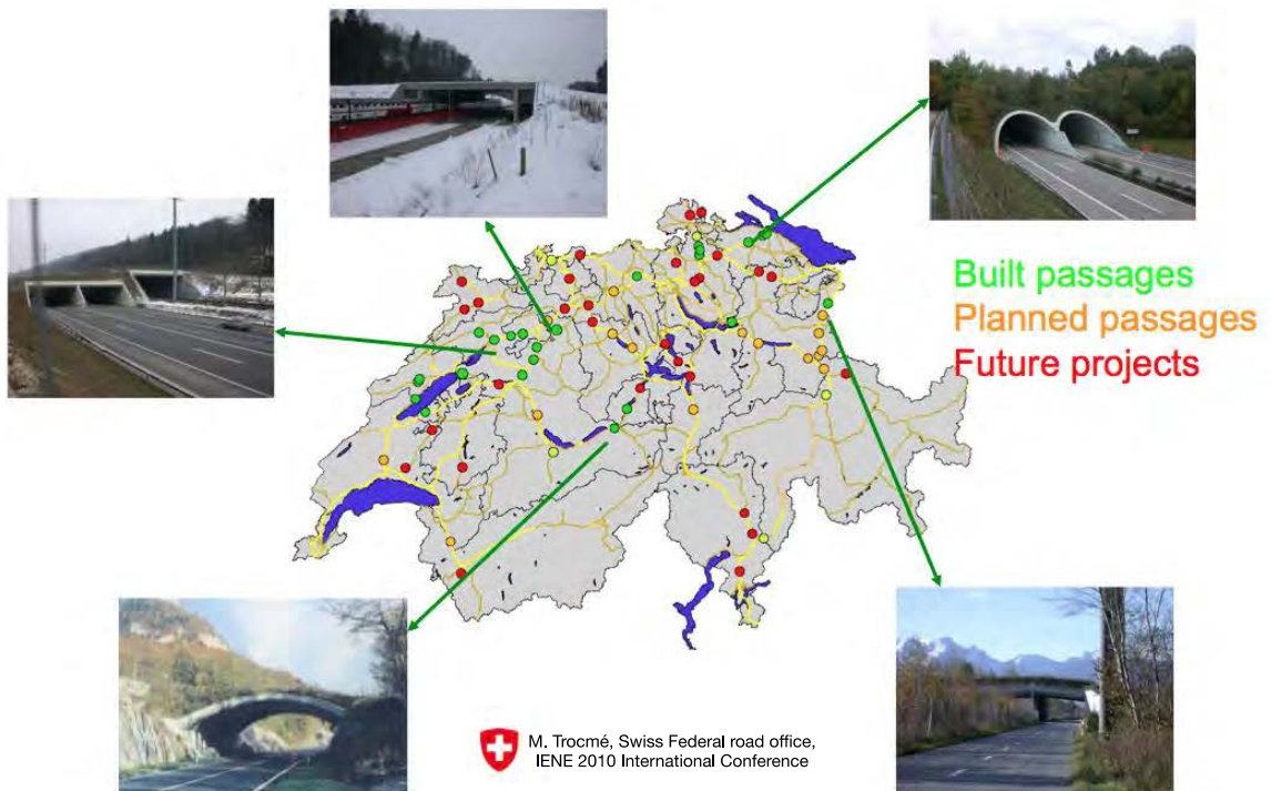
Figur 5. Illustration av befintliga och planerade barriäråtgärder för större däggdjur i Schweiz. Ur: Trocmé (2010)
