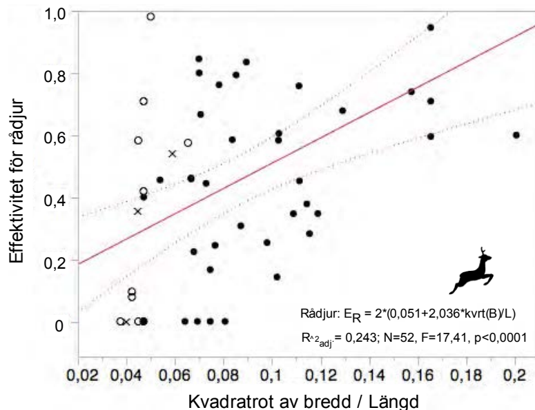
Figur 23. Sambandet mellan passagernas öppenhet, mätt som kvot mellan bredd och längd, och effektiviteten för älg, resp. rådjur. Sambandet skiljer sig något mellan övergångar (öppna cirklar) och undergångar (fyllda cirklar), men i modellen kombineras båda passagertyperna. Källa Seiler & Olsson (under arbete).
