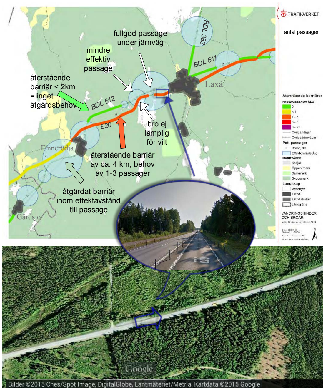
Figur 32. Exempel på resultat-karta efter bristanalysen för älg vid E20 och Västra Stambanan mellan Laxå och Finnerödja. Medan det finns flera mer eller mindre lämpliga passager för älg längs järnvägen saknar E20 nästan helt lämpliga planskilda passagemöjligheter för vilt. Vägen är stängslad och försedd med mitträcke och sidoräcken. Både järnvägen och vägen tillhör de mest viltolycksdrabbade sträckorna i Sverige. Foto: Google Maps och Google StreetView 2014.
