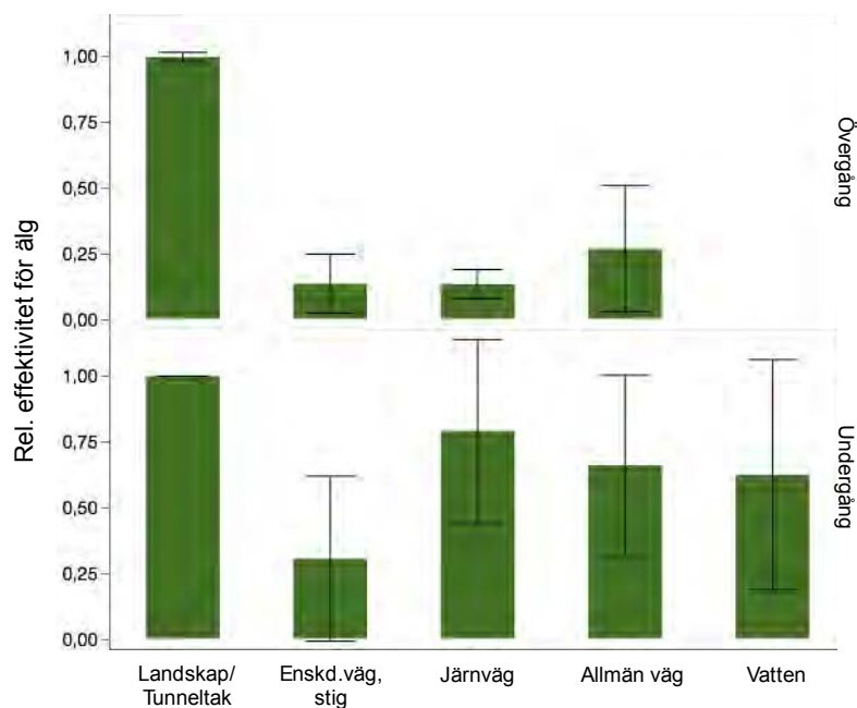
Figur 43. Medelvärden och standardavvikelser i effektivitet för älg av lämpliga passager längs väg- och järnvägsbarriärer.
