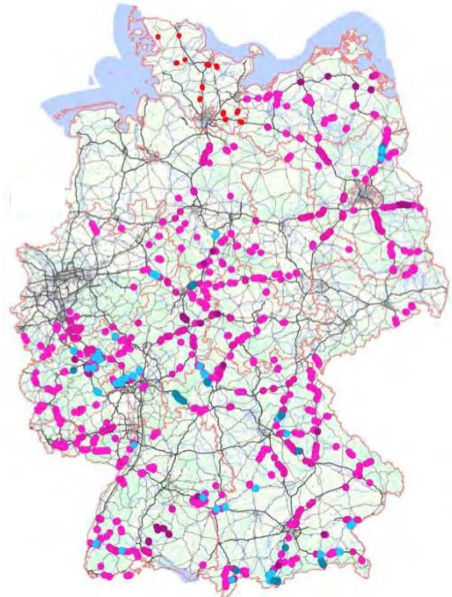
Figur 6. Karta med prioriterade barriäråtgärder där ekologiskt betydelsefulla korridorer skärs av motorvägar och andra transportleder. Ur: Hänel & Reck (2011)
